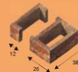
Pustak łupany (słupek)
