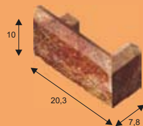
Kształtka łupana
